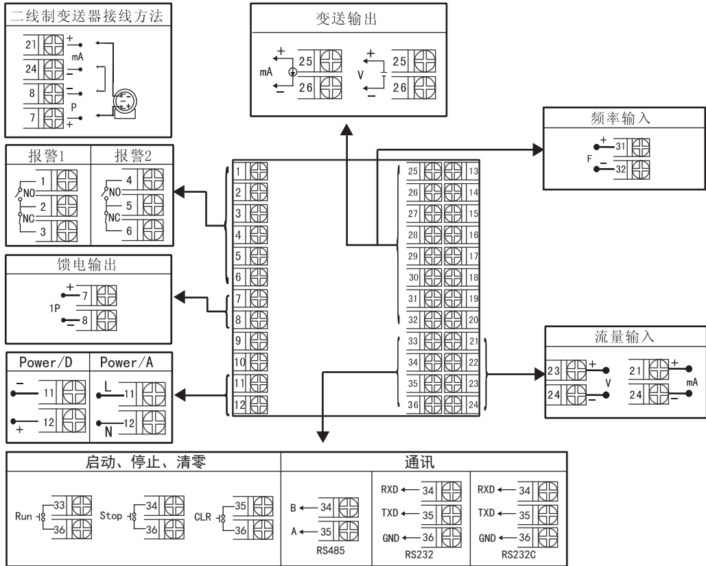
OHR-F602R接线图
