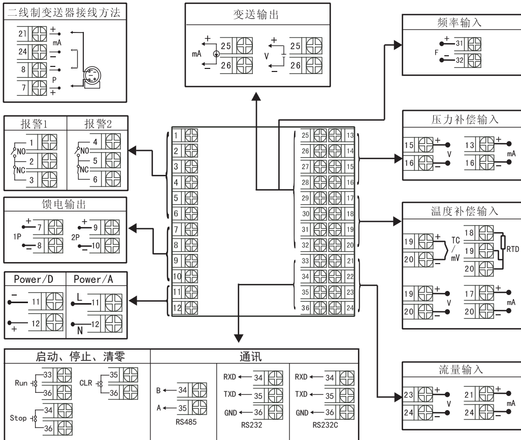
OHR-F602R接线图
