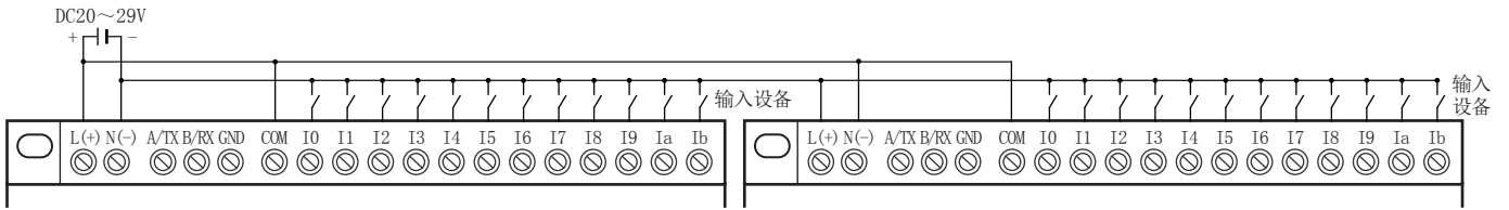
主机和副机连接正公共端子（NPN连接）
