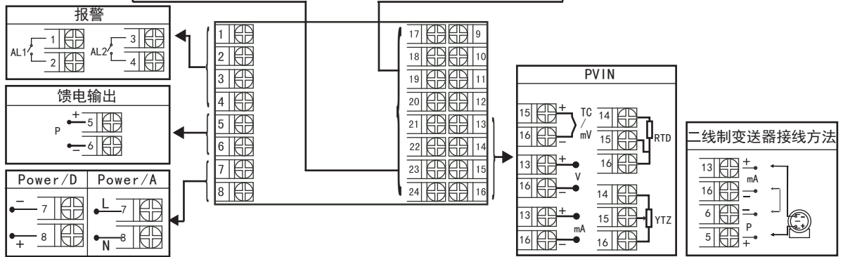
规格尺寸为F型接线图
