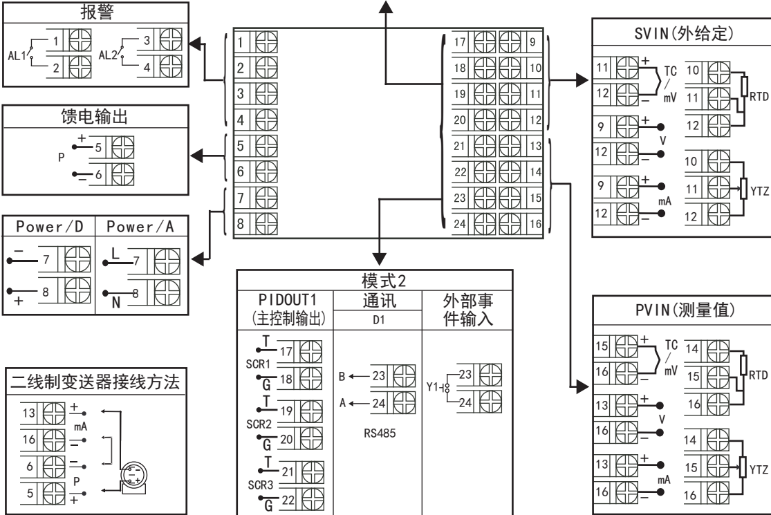
规格尺寸为F型接线图
