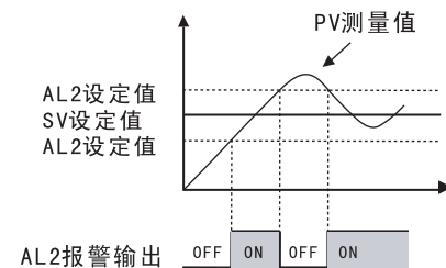
偏差内报警输出
