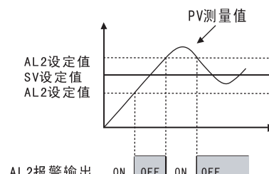
偏差外报警输出
